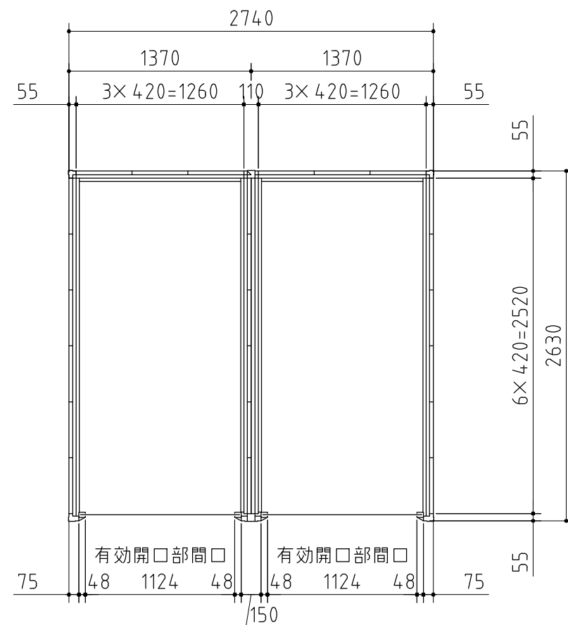
平面図
