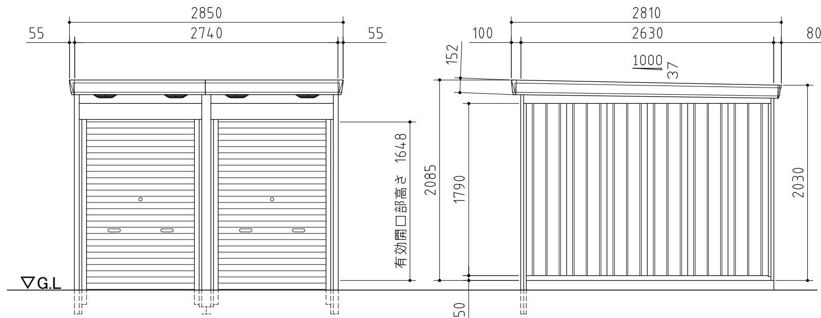
正面図
